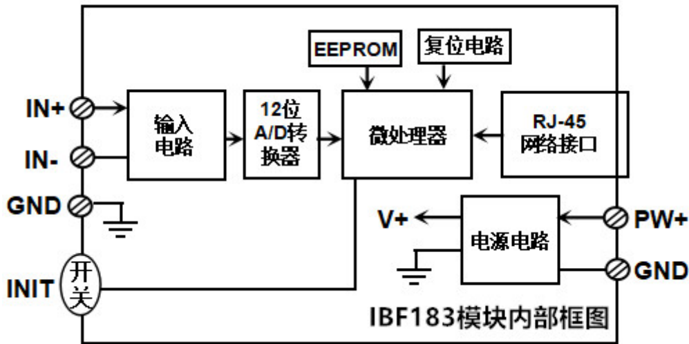
图 2 IBF183 模块内部框图
