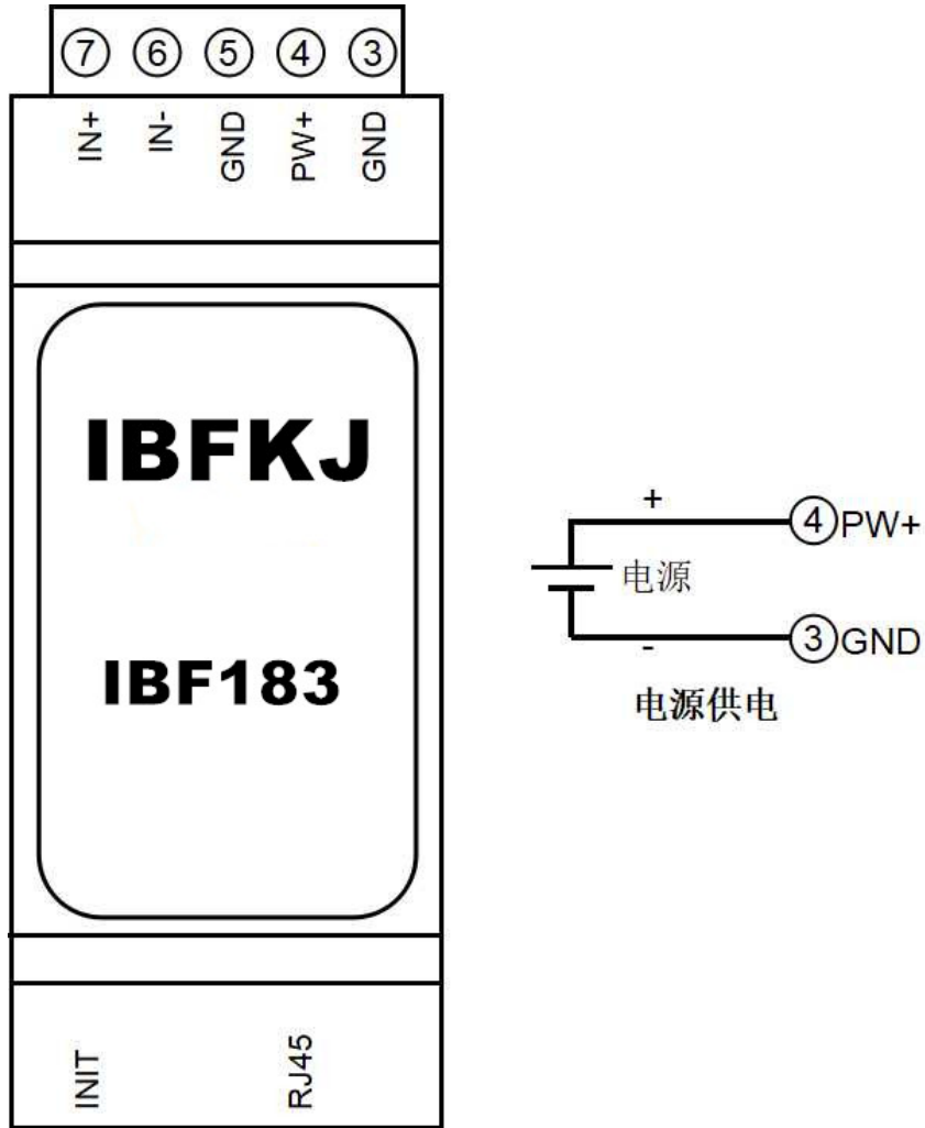
图3 IBF183 模块接线图
